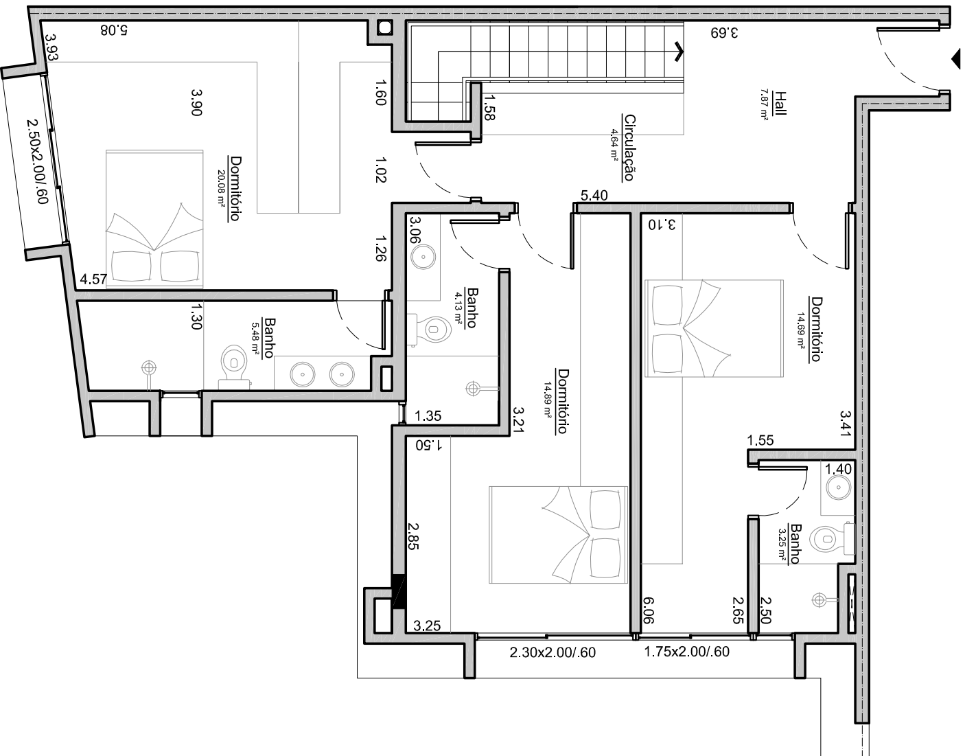
PLANTA BAIXA 3º PAV ÍNTIMO APTO 201
