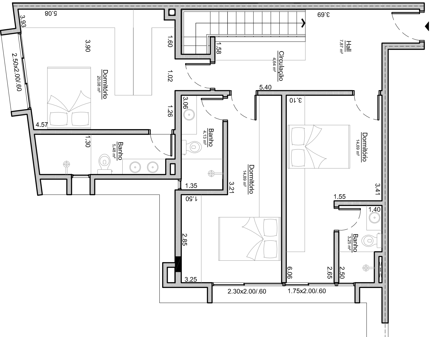
PLANTA BAIXA 4º PAV ÍNTIMO APTO 301
